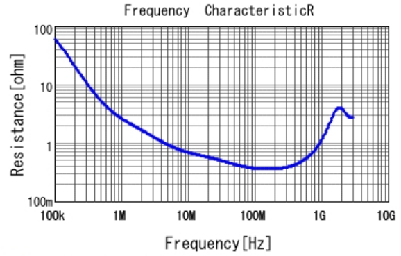
■ GCJ21AR72E102KXJ1 R DCOV, 25degC
