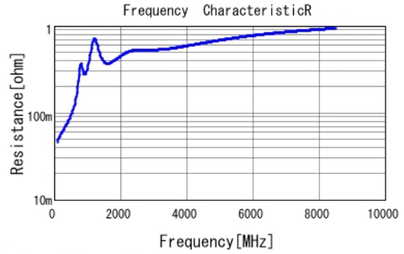
■ GCM1555C1H561FA16 R DCOV, 25degC
