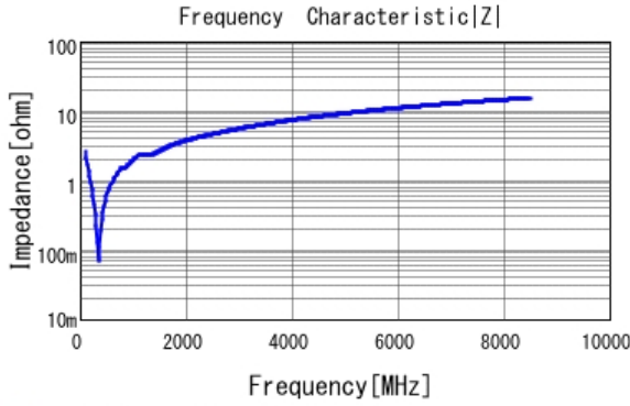
■ GCM1555C1H561FA16 |Z| DCOV, 25degC
