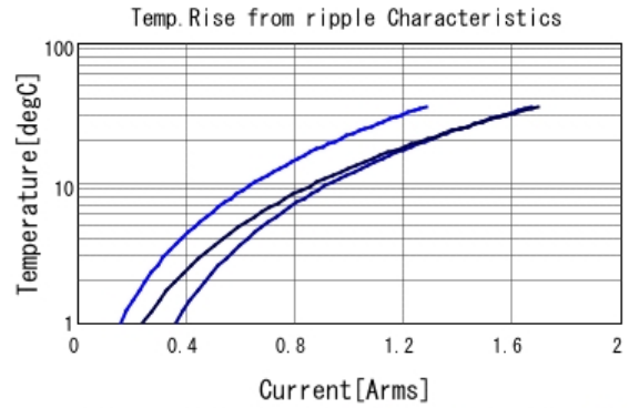
GCM188L81C224KA37 Temp. rise ■ 300kHz ■ 600kHz ■ 1MHz
