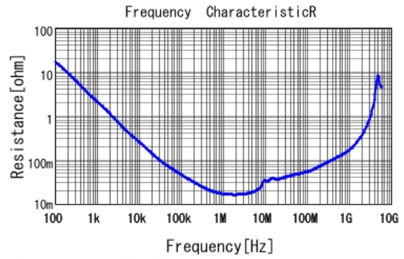
■ GCJ21BR71E225KA01 R DC0V, 25degC
