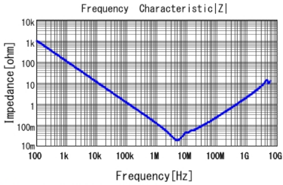
■ GCJ21BR71E225KA01 |Z| DC0V, 25degC
