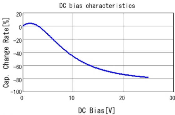
■ GCJ21BR71E225KA01 C-DC bias capchange, 25.0degC, AC1.
