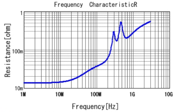
■ GRM21B7U2E272JW32 R DCOV, 25degC
