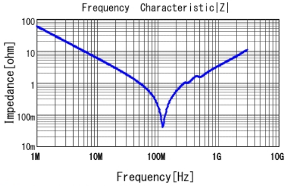
■ GRM21B7U2E272JW32 |Z| DCOV, 25degC
