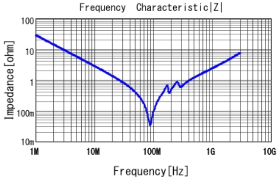
■ GRM21B7U2E562JW32 |Z| DCOV, 25degC
