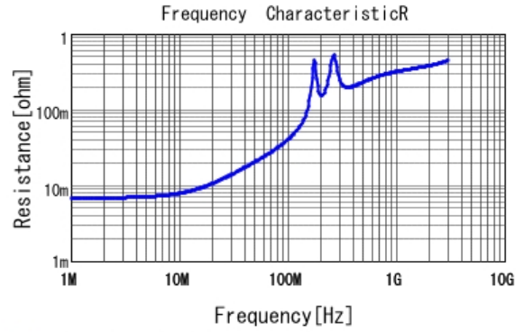
■ GRM21B7U2E562JW32 R DCOV, 25degC
