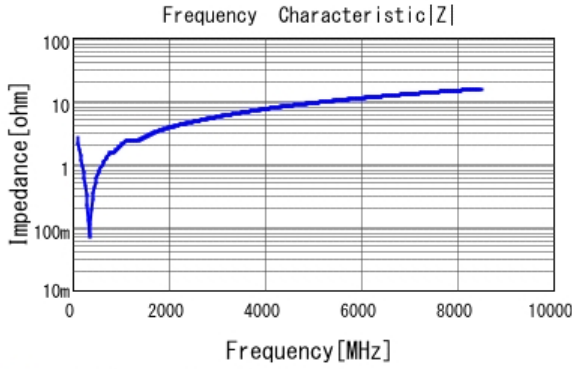
■ GCM1555C1H561JA16 |Z| DCOV, 25degC
