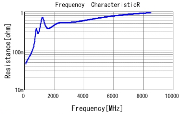
■ GCM1555C1H561JA16 R DCOV, 25degC
