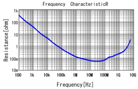
GCM155R71E223KA55 R DCOV, 25degC
