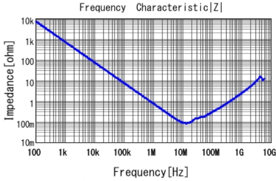
■ GCJ21BR71H224KA01 |Z| DC0V, 25degC
