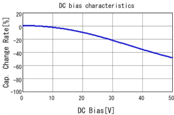
■ GCJ21BR71H224KA01 C-DC bias capchange, 25.0degC, AC1.
