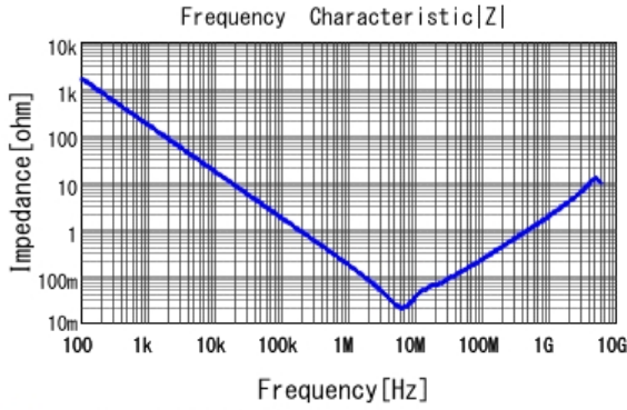
■ GCJ219R71C105KA01 |Z| DC0V, 25degC
