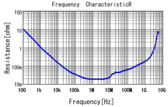
■ GCJ219R71C105KA01 R DC0V, 25degC
