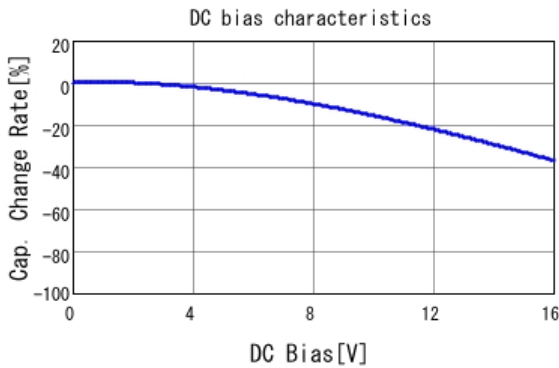
■ GCJ219R71C105KA01 C-DC bias capchange, 25.0degC, AC1.
