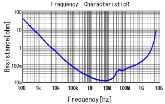
■ GRM188R71E224KA88 R DCOV, 25degC
