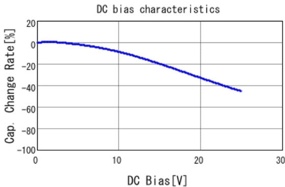
■ GRM188R71E224KA88 C-DC bias capchange, 25.0degC, AC1.
