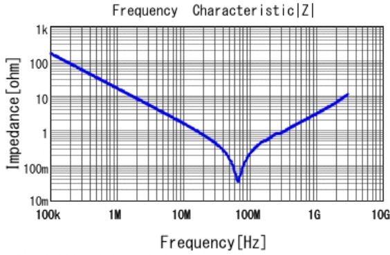
■ GC321AD72E103KX01 |Z| DC0V, 25degC
