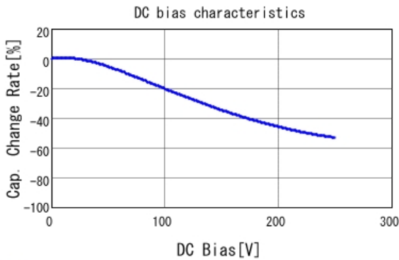
■ GC321AD72E103KX01 C-DC bias capchange, 25.0degC, AC1V
