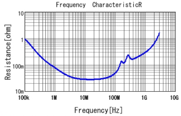
■ GC321AD72E103KX01 R DC0V, 25degC
