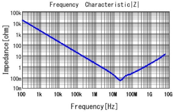
■ GCJ188R71E104KA12 |Z| DCOV, 25degC
