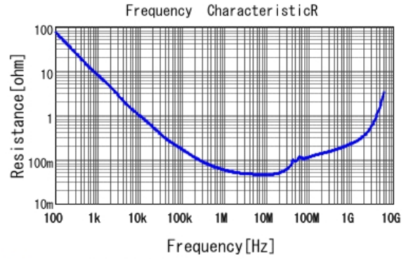
■ GCJ188R71E104KA12 R DCOV, 25degC
