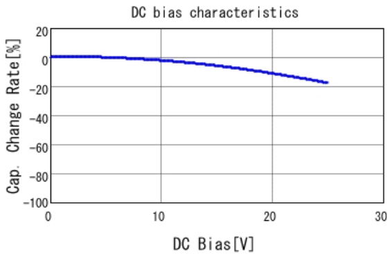
■ GCJ188R71E104KA12 C-DC bias capchange, 25.0degC, AC1.
