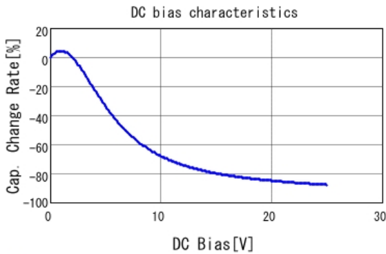
■ GRT155R61E224KE01 C-DC bias capchange, 25.0degC, AC1.
