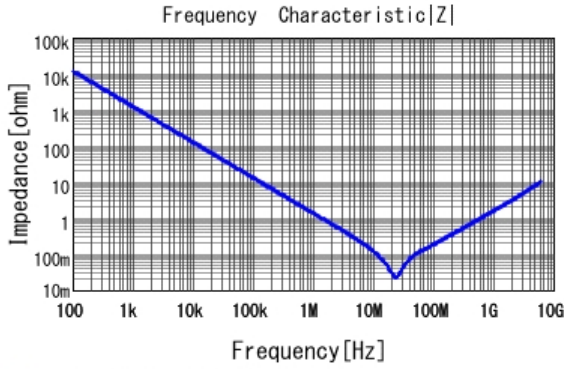
■ GRT155R61E224KE01 |Z| DC0V, 25degC
