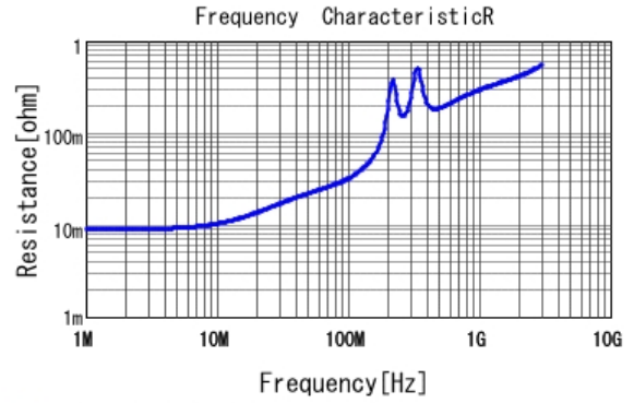
■ GRM21B7U2E392JW32 R DCOV, 25degC
