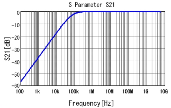
■ GCJ188R71E223KA01 S21 DC0V, 25degC
