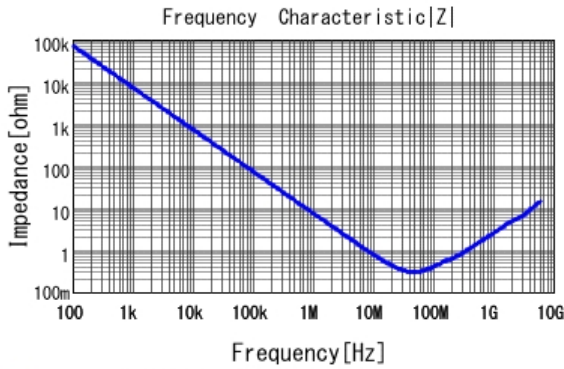
■ GCJ188R71E223KA01 |Z| DCOV, 25degC
