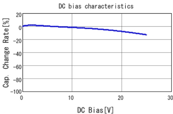
■ GCJ188R71E223KA01 C-DC bias capchange, 25.0degC, AC1.
