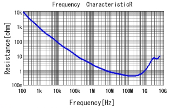
■ GCJ188R71E102KA01 R DCOV, 25degC
