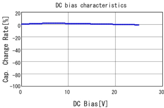
■ GCJ188R71E102KA01 C-DC bias capchange, 25.0degC, AC1.
