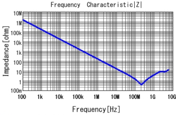
■ GCJ188R71E102KA01 |Z| DCOV, 25degC
