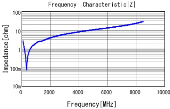
■ GRM1555C1H561JA01 |Z| DCOV, 25degC
