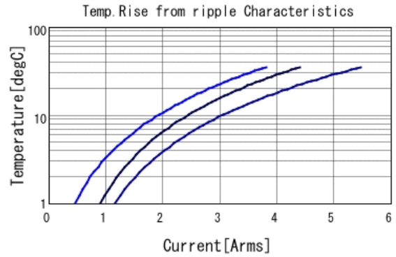
GCM21BC7YA475KE36 Temp. rise ■ 100kHz ■ 500kHz ■ 1MHz
