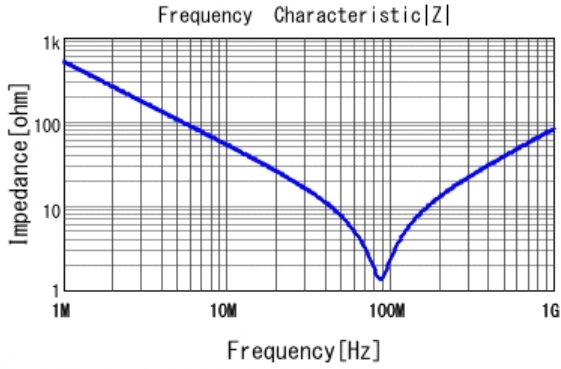
■ DE1B3RA331KA4BQ01F |Z| DCOV, 20degC
