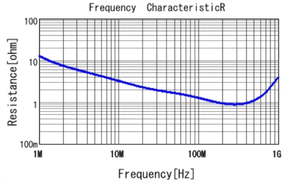
■ DE1B3RA331KA4BQ01F R DCOV, 20degC
