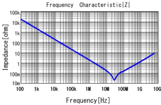
■ GRM155R71H104KE14 |Z| DC0V, 25degC
