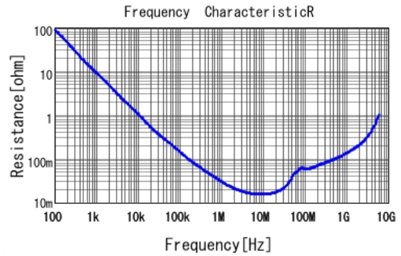
■ GRM155R71H104KE14 R DC0V, 25degC
