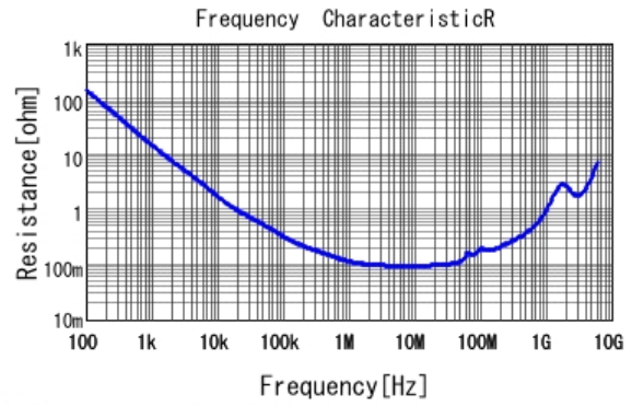
■ GCJ21BR72A473KA01 R DCOV, 25degC
