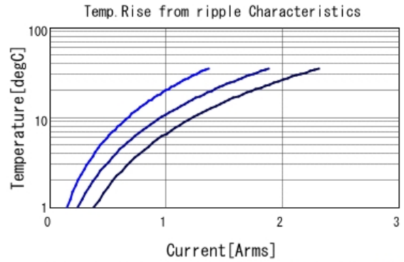
GCJ188R91E474KA01 Temp. rise ■ 200kHz ■ 500kHz ■ 1MHz
