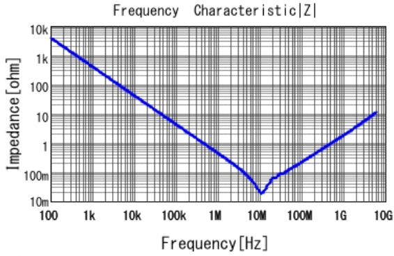
■ GCJ188R91E474KA01 |Z| DCOV, 25degC
