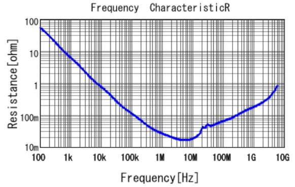
■ GCJ188R91E474KA01 R DCOV, 25degC
