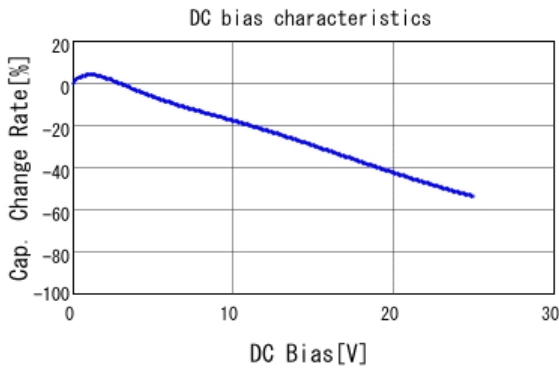
■ GCJ188R91E474KA01 C-DC bias capchange, 25.0degC, AC1.
