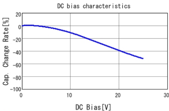
GCM21BR71E684KA55 C-DC bias capchange, 25.0degC, AC1.
