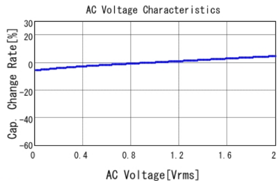
GCM21BR71E684KA55 C-AC Voltage capchange, DCOV, 25.0d
