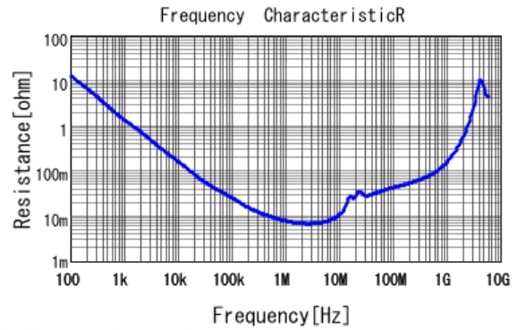
GCM21BR71E684KA55 R DCOV, 25degC
