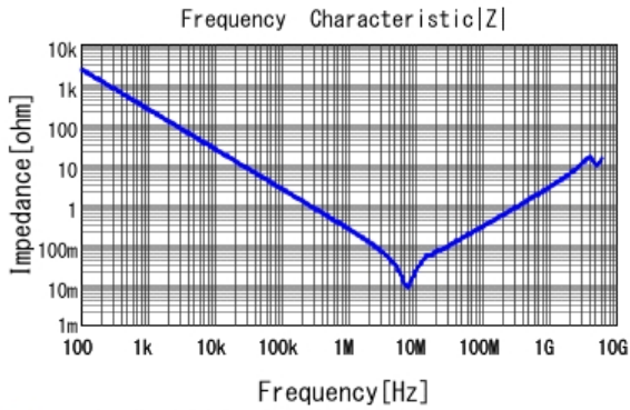
GCM21BR71E684KA55 |Z| DCOV, 25degC
