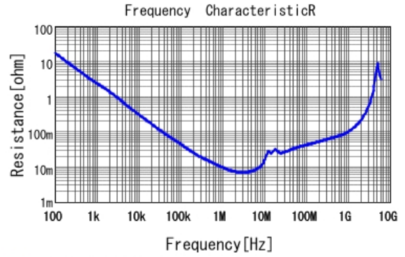
GCM21BR71E155KA54 R DC0V, 25degC
