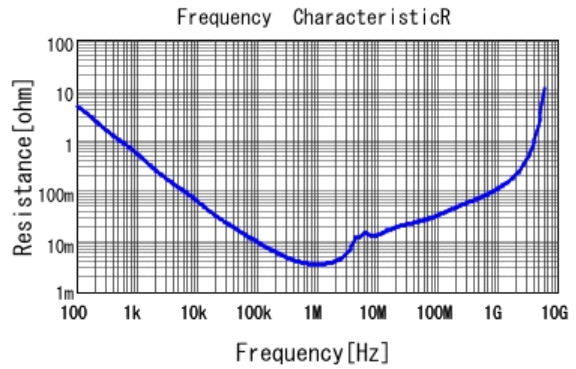
■ GCM21BR70J106KE22 R DCOV, 25degC
