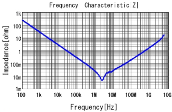
■ GCM21BR70J106KE22 |Z| DCOV, 25degC
