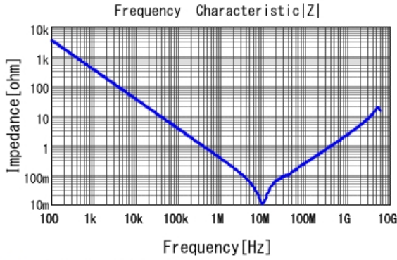
GCM219R71E474KA55 |Z| DCOV, 25degC
