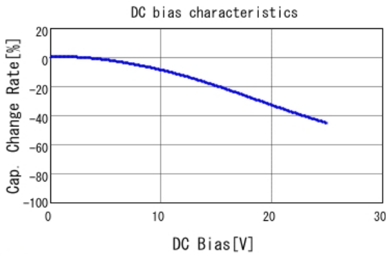
GCM219R71E474KA55 C-DC bias capchange, 25.0degC, AC1.
