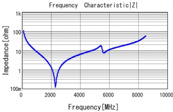
■ GCQ1555C1H150FB01 |Z| DC0V, 25degC
