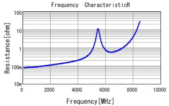
■ GCQ1555C1H150FB01 R DC0V, 25degC
