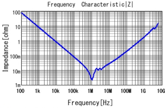
GCM32EC71E226KE36 |Z| DC0V, 25degC
