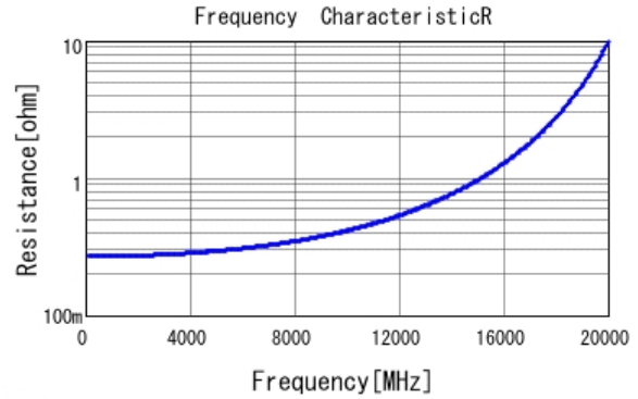
■ GCQ1555C1HR80WB01 R DC0V, 25degC
