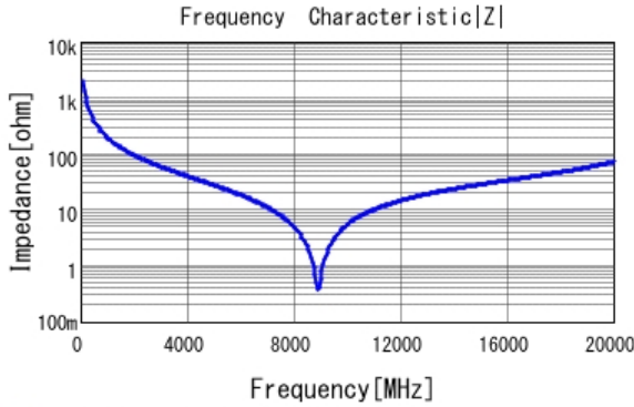
■ GCQ1555C1HR80WB01 |Z| DC0V, 25degC
