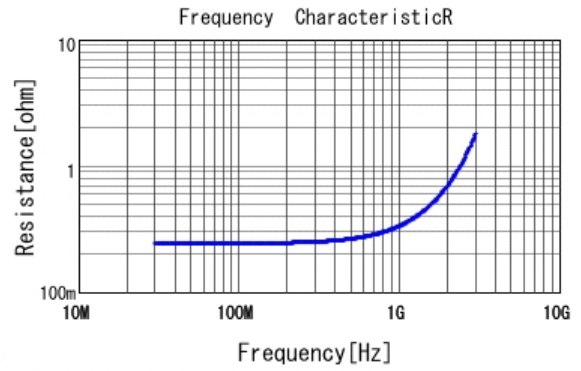
■ RCE5C3A270J2M1H03A R DCOV, 25degC
