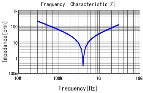
■ RCE5C3A270J2M1H03A |Z| DCOV, 25degC
