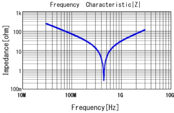
■ RCE5C3A220J2M1H03A |Z| DCOV, 25degC
