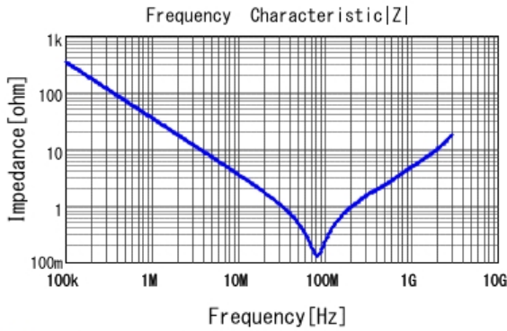
■ GCJ31BR73A472KXJ1 |Z| DC0V, 25degC
