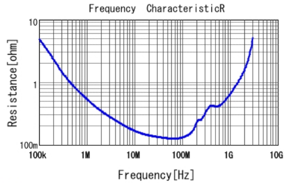
■ GCJ31BR73A472KXJ1 R DC0V, 25degC
