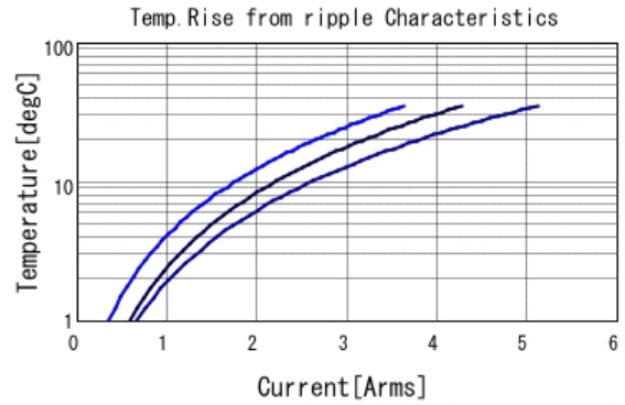
GRM21BC7YA475KE11 Temp. rise ■ 100kHz ■ 500kHz ■ 1MHz
