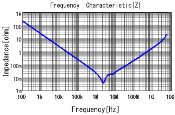
■ GRM21BC71C106KE11 |Z| DCOV, 25degC
