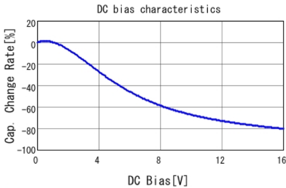
■ GRM21BC71C106KE11 C-DC bias capchange, 25.0degC, AC1V
