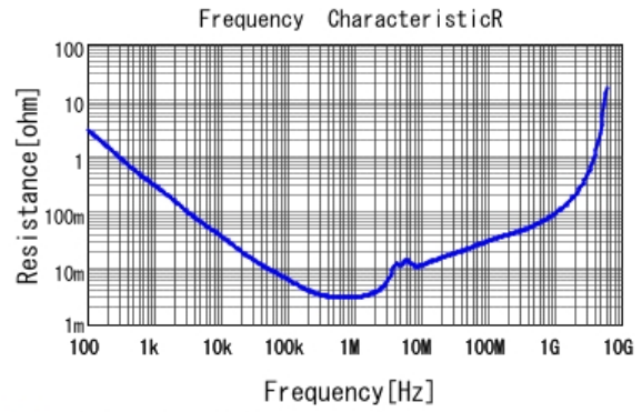
■ GRM21BC71C106KE11 R DCOV, 25degC
