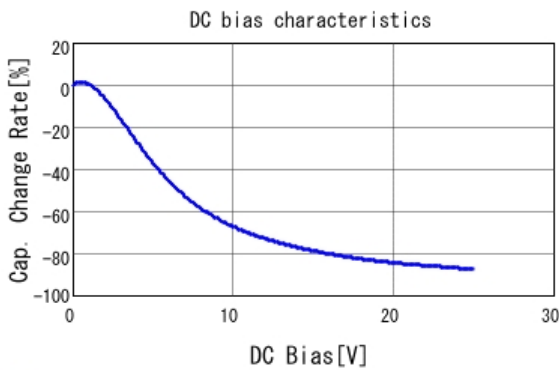
■ GRM21BC71E106KE11 C-DC bias capchange, 25.0degC, AC1V
