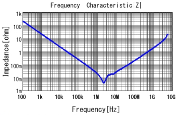
■ GRM21BC71E106KE11 |Z| DC0V, 25degC
