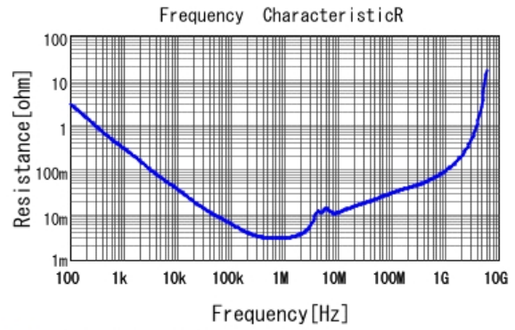
■ GRM21BC71E106KE11 R DC0V, 25degC
