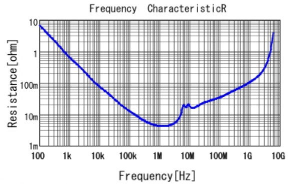
■ GRM21BC71E475KE11 R DCOV, 25degC
