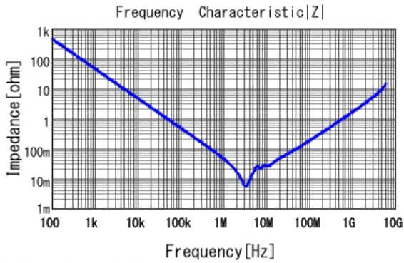
■ GRM21BC71E475KE11 |Z| DCOV, 25degC
