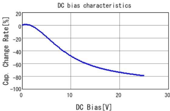
■ GRM21BC71E475KE11 C-DC bias capchange, 25.0degC, AC1V
