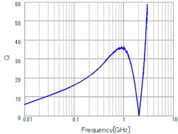
LQG15WH47NH02 Q.
