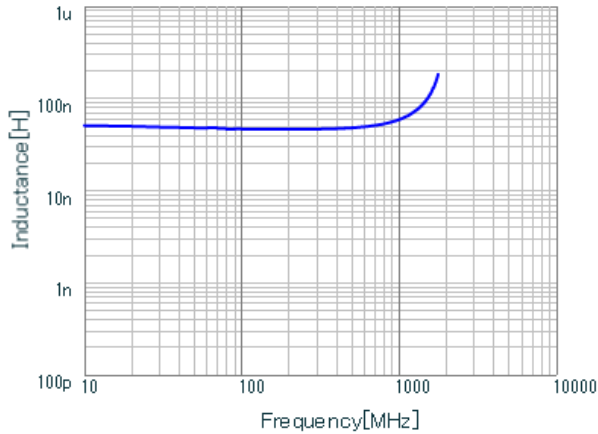
LQG15WH47NH02 L.
