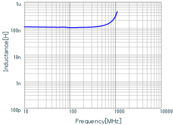
LQG15WZR11J02 L.
