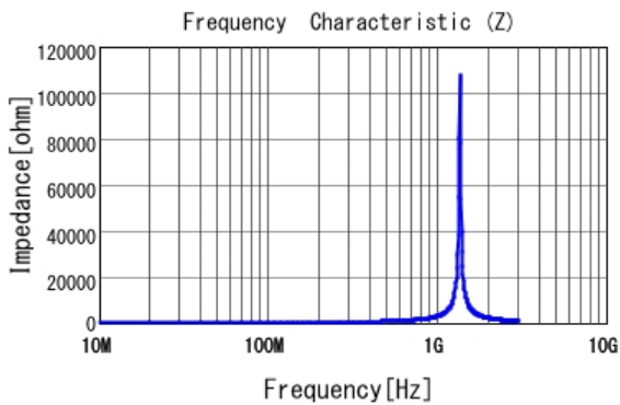
■ LQW18ASR22G0C |Z|
