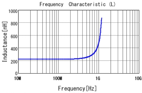
■ LQW18ASR22G0C L
