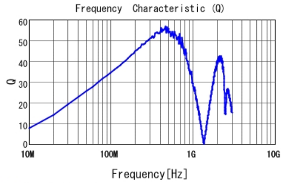
■ LQW18ASR22G0C Q
