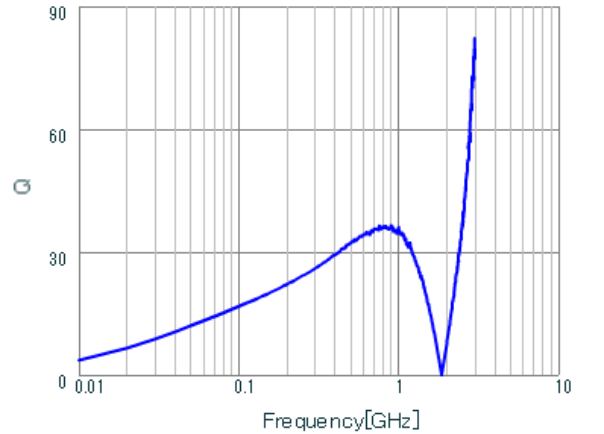
LQG15WH56NH02 Q.
