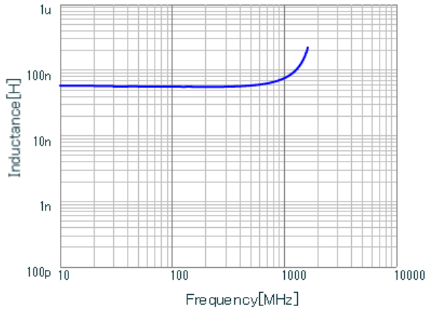
LQG15WH56NH02 L.
