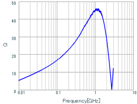
LQG15WZ27NH02 Q.
