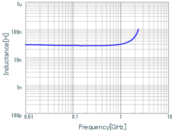
LQG15WZ27NH02 L.
