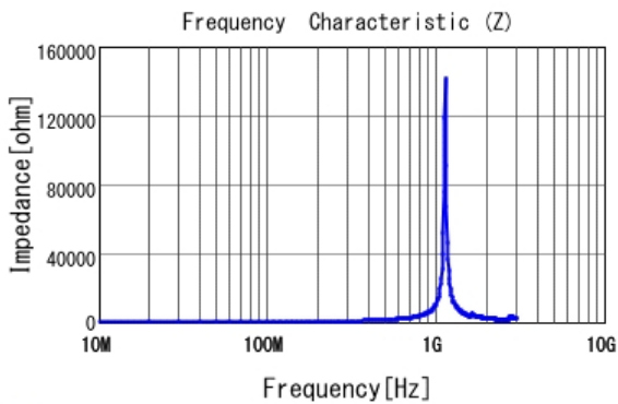
■ LQW18ASR39G0C |Z|
