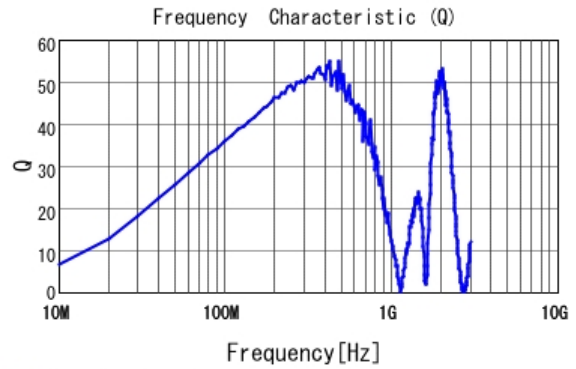
■ LQW18ASR39G0C Q
