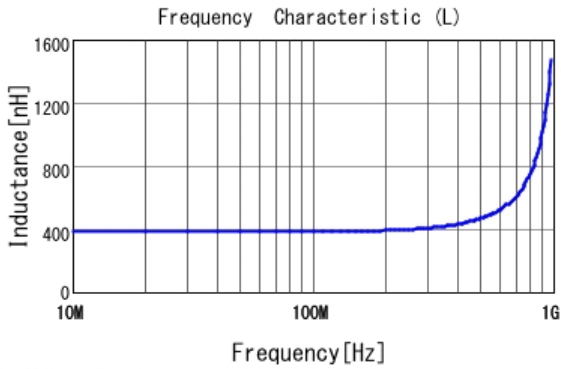
■ LQW18ASR39G0C L
