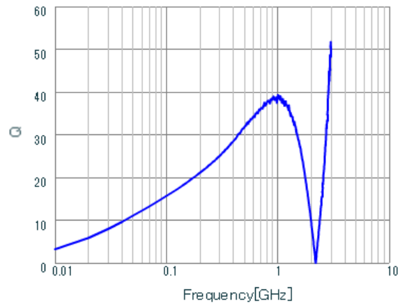
LQG15WH43NH02 Q.
