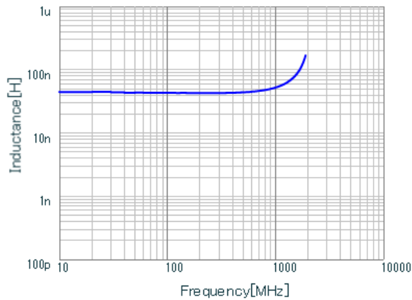
LQG15WH43NH02 L.
