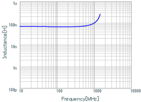
LQG15WH68NG02 L.
