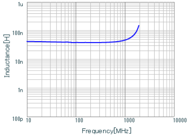
LQG15WZ39NG02 L.
