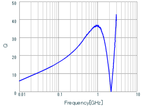
LQG15WZ39NG02 Q.
