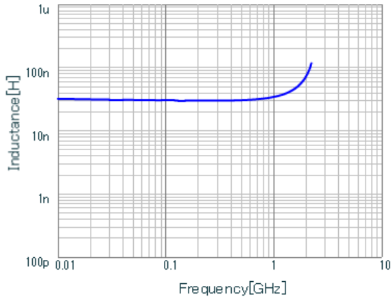
LQG15WZ30NJ02 L.
