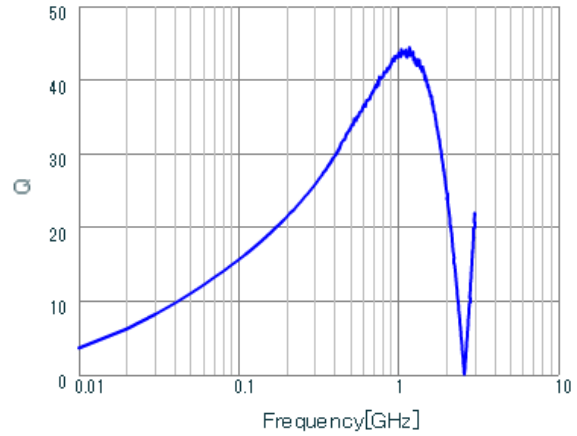
LQG15WZ30NJ02 Q.
