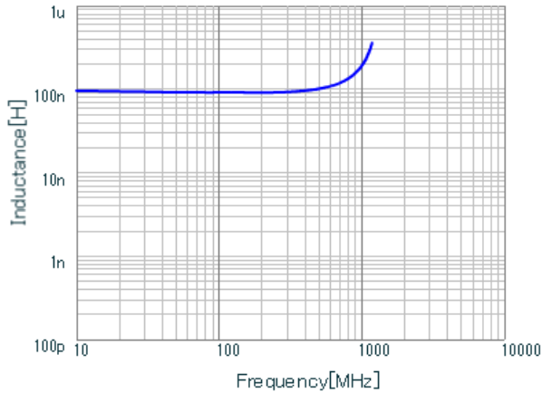
LQG15WH91NG02 L.
