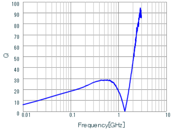
LQG15WH91NG02 Q.
