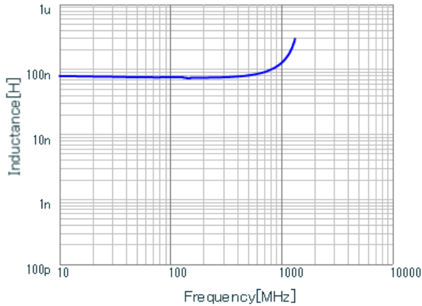
LQG15WH75NG02 L.
