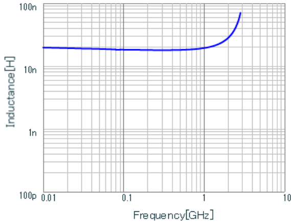
LQG15WH18NG02 L.
