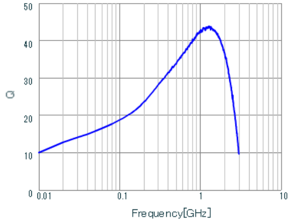
LQG15WH18NG02 Q.
